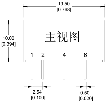
封装尺寸图
